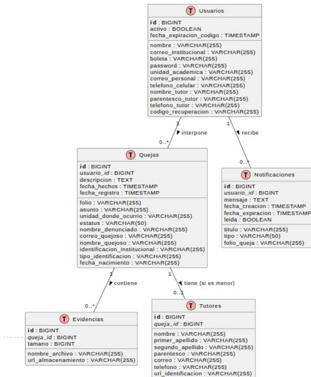
Figura 4.4: Modelo entidad-relación del microservicio de atención al quejoso
