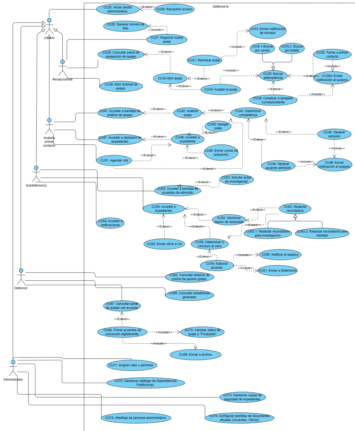
Figura 4.3: Diagrama de casos de uso del microservicio de atención al quejoso
