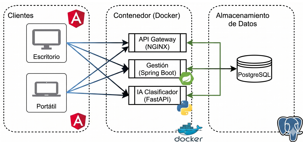
Figura 3.1: Arquitectura general propuesta para la plataforma institucional.
