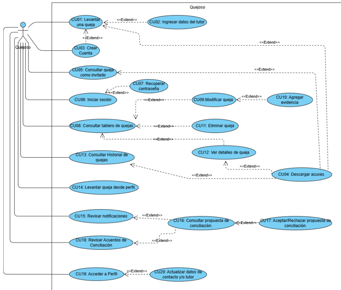
Figura 4.2: Diagrama de casos de uso del microservicio de atención al quejoso
