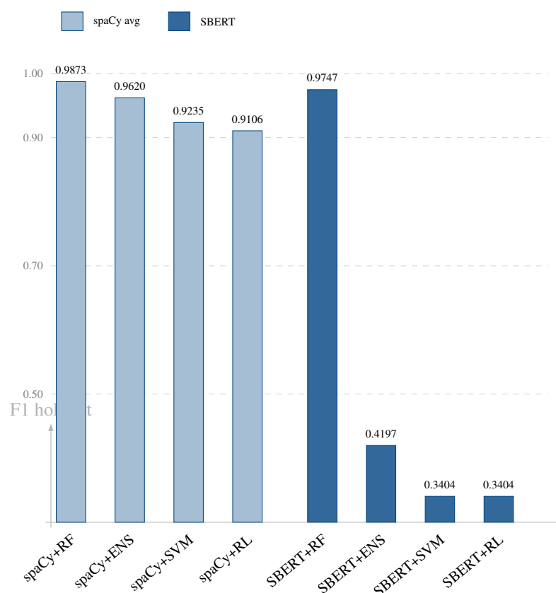
Figura 4.8: F1 ponderado en holdout por combinación de modelo (evaluación sin atributos jurídicos)
