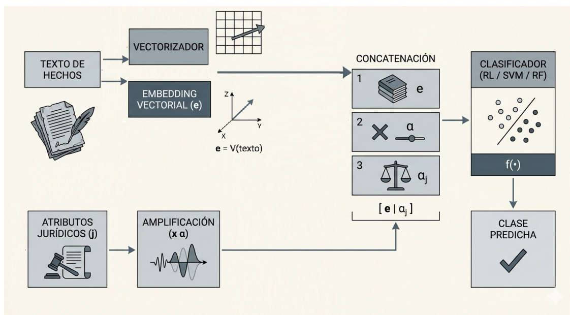
Figura 4.7: Arquitectura del pipeline de clasificación combinado
